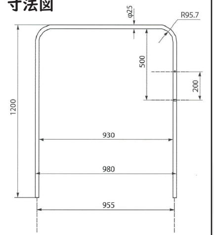
寸法図
