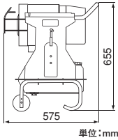
◀ 段積み収納
