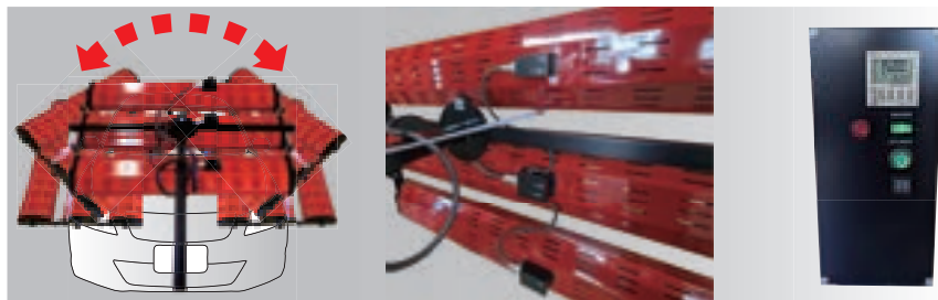
▲バンクが 180 度回転 ▲バンクごとに ON/OFF スイッチ ▲デジタルタイマー
